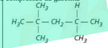
isooctano
