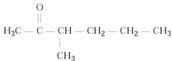
3-metil-2-hexanona
